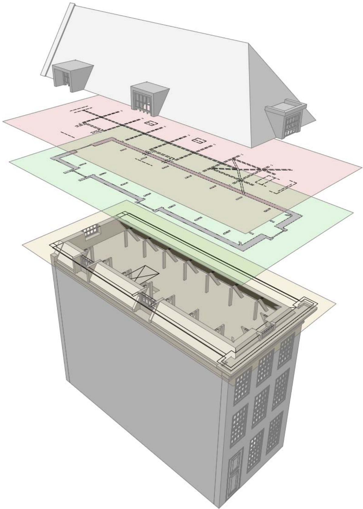
Figuur 3: projectievlak aangebracht: lichtgeel vlak voor componentaanzicht, lichtgroen voor componentdoorsnijing, roze voor componentprojectie.
