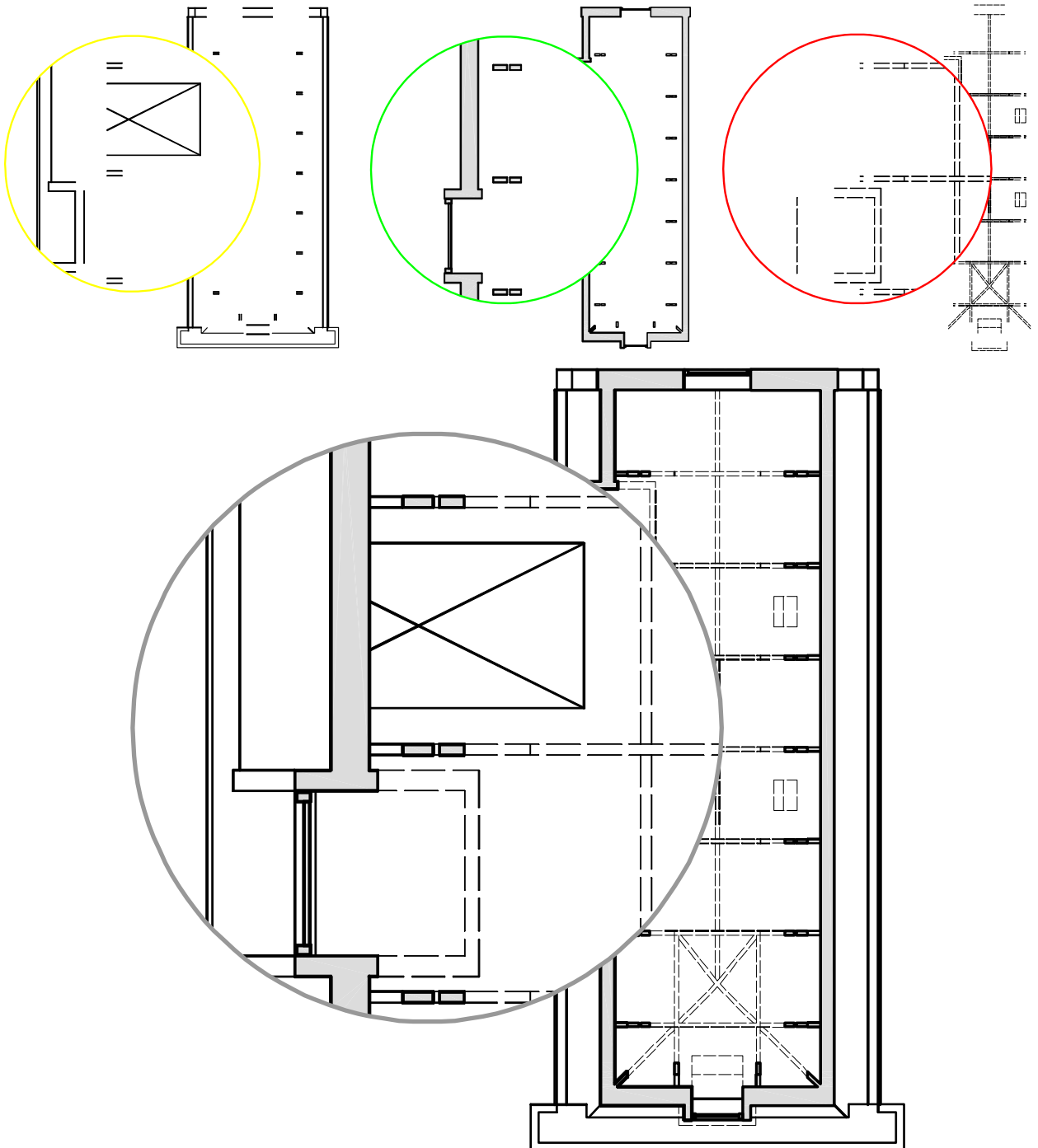
Figuur 4: componentaanzicht (binnen gele uitsnede), componentdoorsnijding (groene uitsnede) en componentprojectie (rode uitsnede) gesuperposeerd in één 2D-plattegrond (binnen grijze uitsnede).
